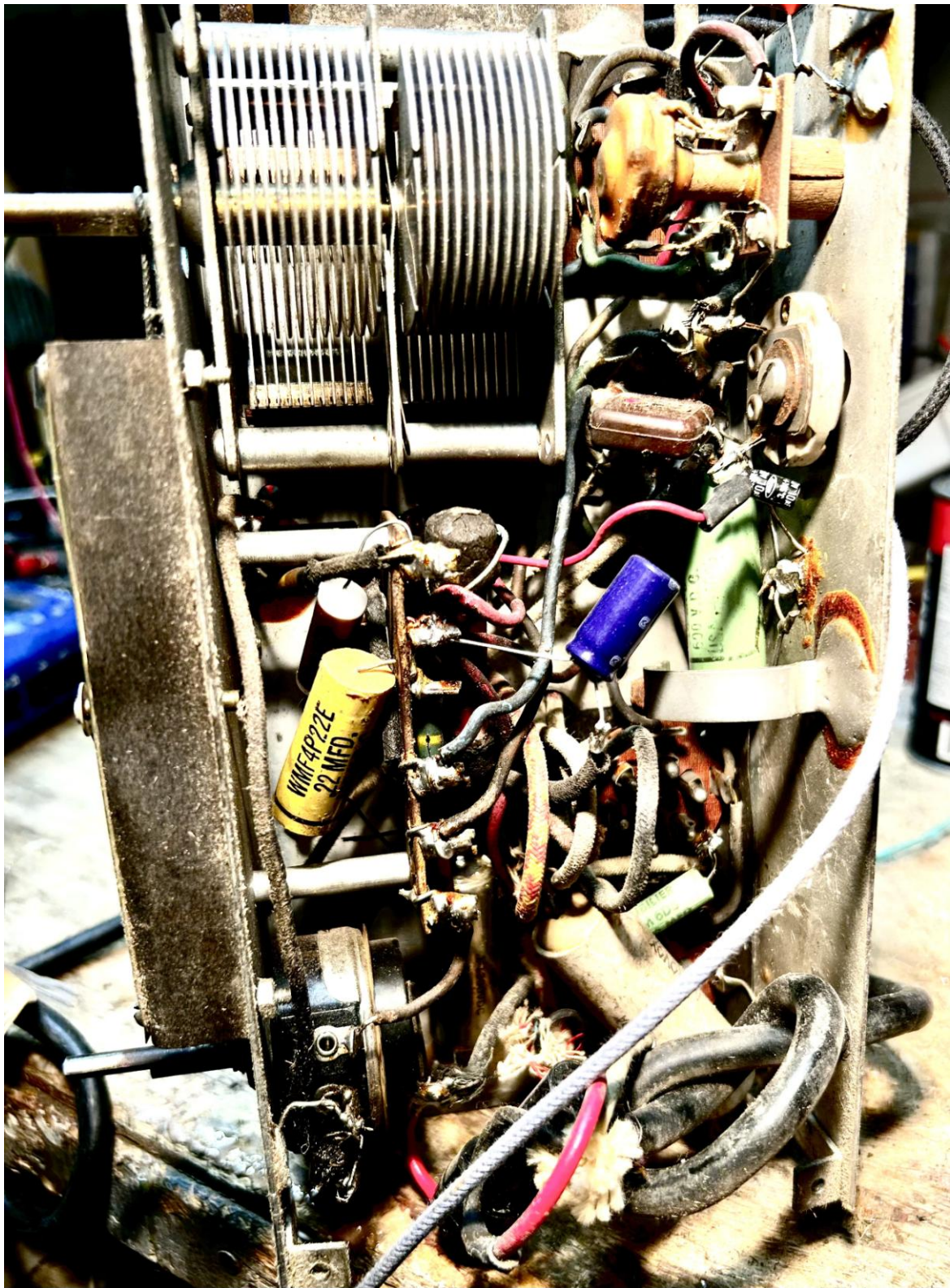
Les condensateurs ont été changés. Les résistances <dogbone> était encore bonne condition.
